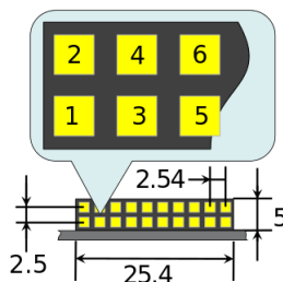
Рис. 4.6: Размеры и нумерация выводов в разьеме ВРС (BackPlane Connector), вид со стороны разъема
