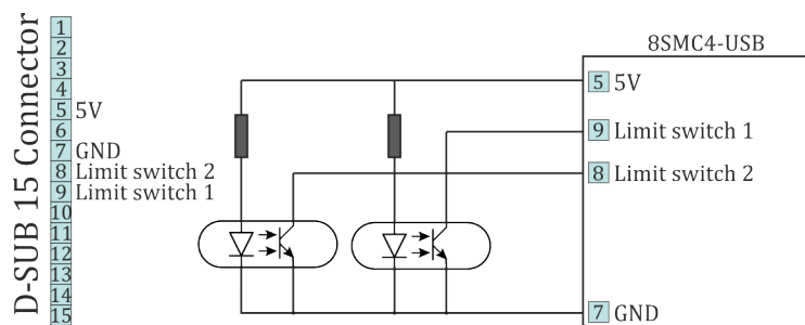
Рис. 4.30: Подключение концевиков типа «оптопара»
