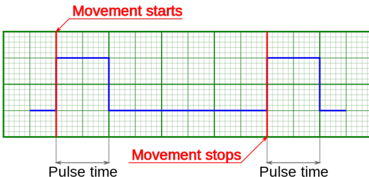
Рис. 4.56: Выходные импульсы синхронизации при генерации их на старте и на остановке движения (импульс фиксированной длительности)
