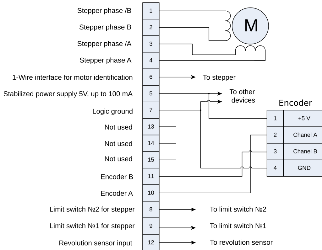
Рис. 3.14: Общая схема подключения позиционера с энкодером через разъем D-sub
