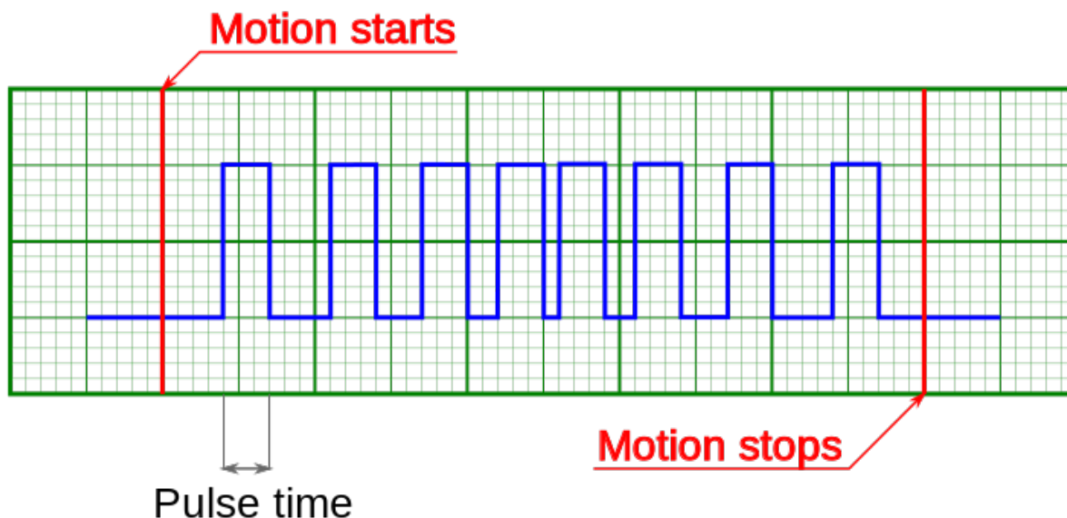
Рис. 4.59: Выходные импульсы синхронизации при движении с ускорением и генерации импульсов каждое смещение на заданное расстояние (импульс измеряется в микросекундах)
