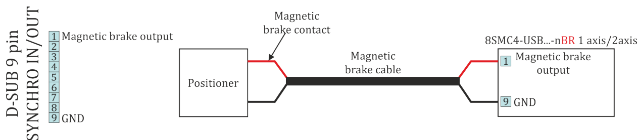
Рис. 4.42: Схема подключения магнитного тормоза к одноосной или двухосной системе
