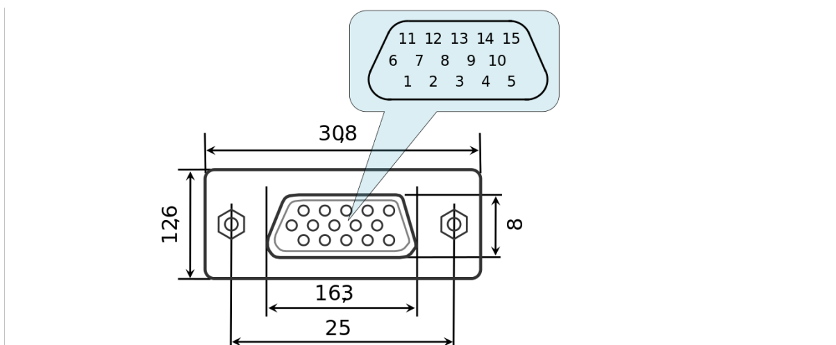
Рис. 4.11: Размеры и нумерация выводов в разъеме DSub, вид спереди
