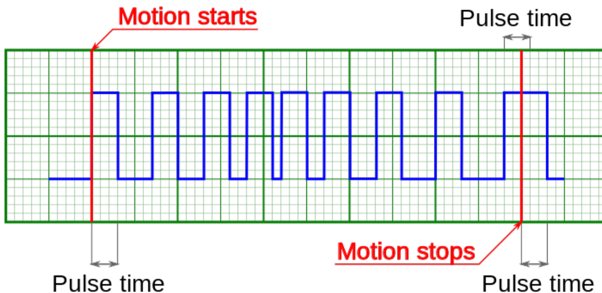
Рис. 4.60: Иллюстрация наложения импульсов синхронизации по старту и по остановке движения смещение на заданное расстояние (длительность импульса, измеренная в микросекундах)
