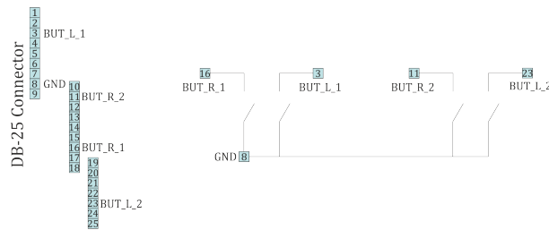
Рис. 4.49: Типовая схема подключения кнопок к разъёму многоосной системы
