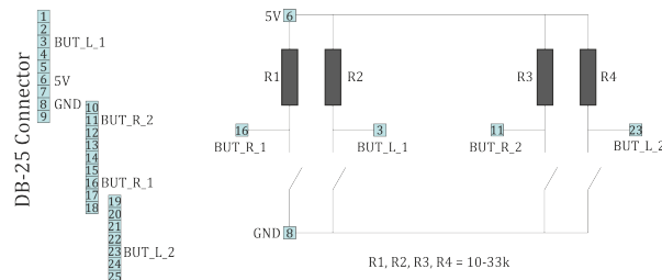
Рис. 4.50: Схема подключения кнопок к разъёму многоосной системы для старых модулей версии 1.1 и ниже
