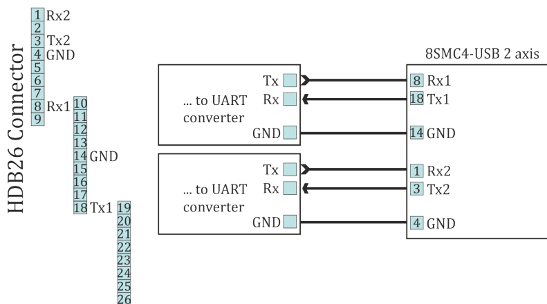
Рис. 4.72: Рекомендуемая схема подключения для двухосной системы
