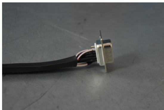
Рис. 3.18: Готовый провод, идущий от мотора с D-SUB разъёмом на конце
