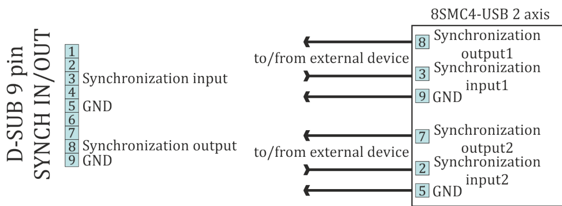
Рис. 4.63: Схема подключения к каналам синхронизации на двухосной системе
