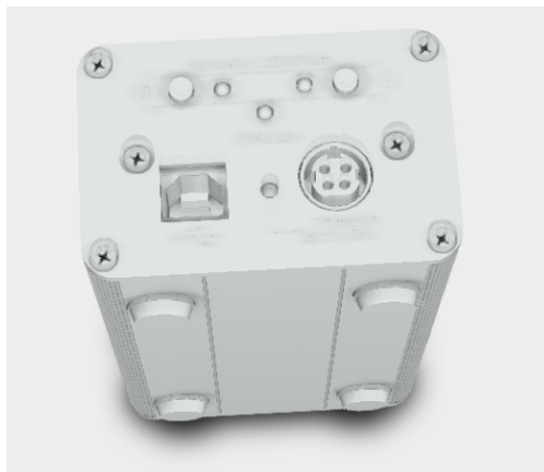
Рис. 4.9: Контроллер в металлическом корпусе, одноосный вариант 3D (модель 8SMC4-USB-B8-1)
