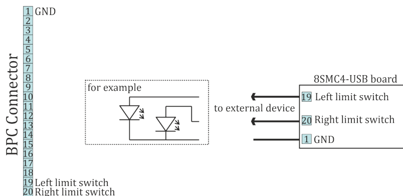
Рис. 4.39: Схема подключения индикаторов концевых выключателей к плате контроллера
