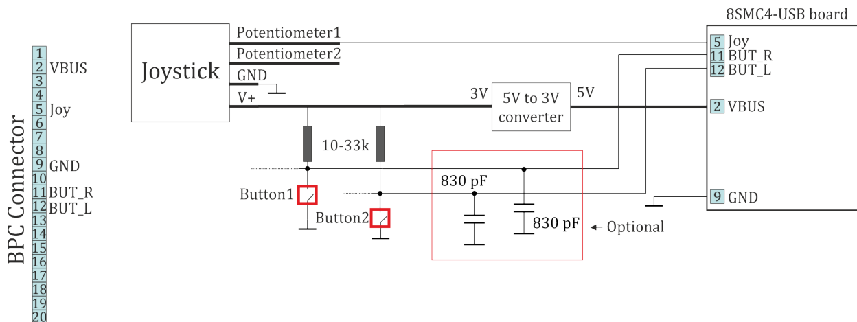
Рис. 4.44: Схема подключения джойстика к плате контроллера через разъём ВРС
