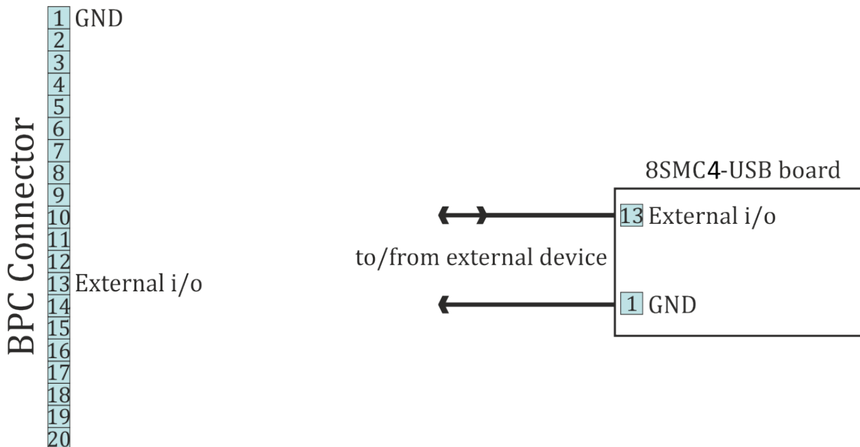
Рис. 4.66: Схема подключения к цифровому входу выходу на плате контроллера
