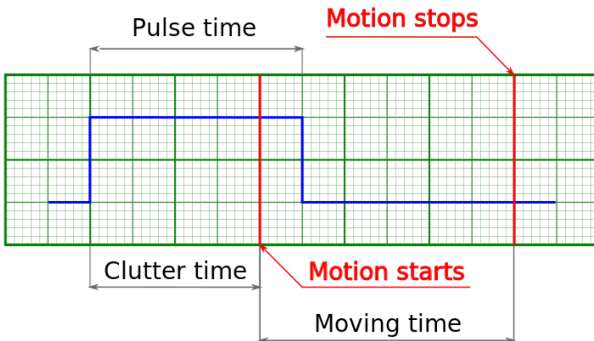
Рис. 4.52: Движение начнётся раз входной импульс дольше времени подавления дребезга
