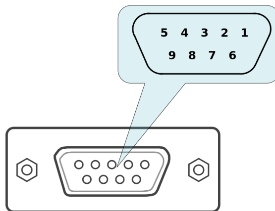
Рис. 4.22: Размеры и нумерация выводов в разъеме DSub, вид спереди
