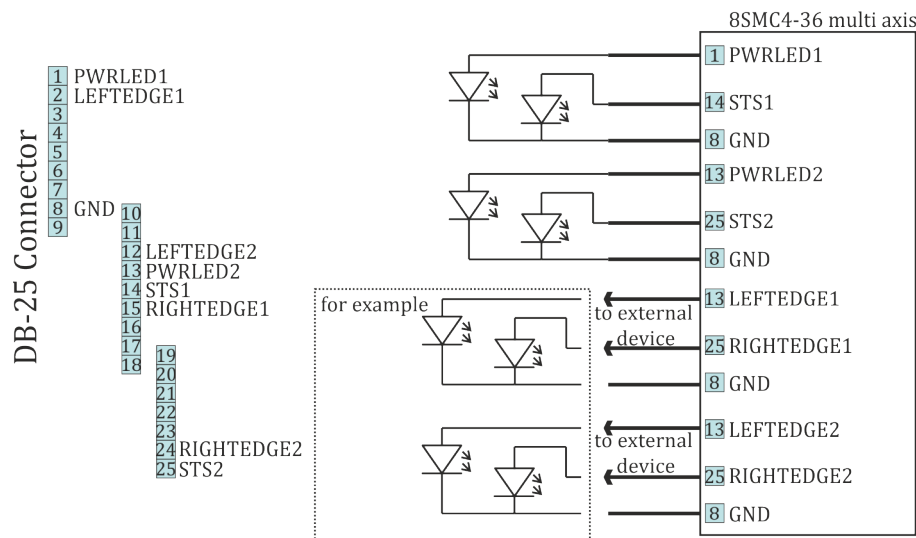
Рис. 4.40: Схема подключения индикаторов Power и Status к плате контроллера
