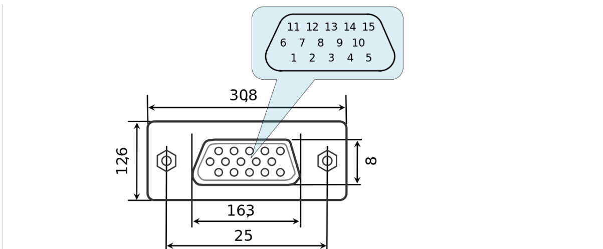
Рис. 4.2: Размеры и нумерация выводов в разъеме DSub, вид спереди
