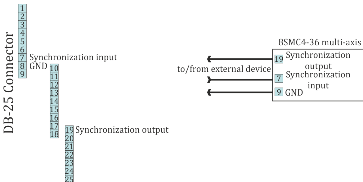
Рис. 4.64: Схема подключения к каналам синхронизации в многоосной системе
