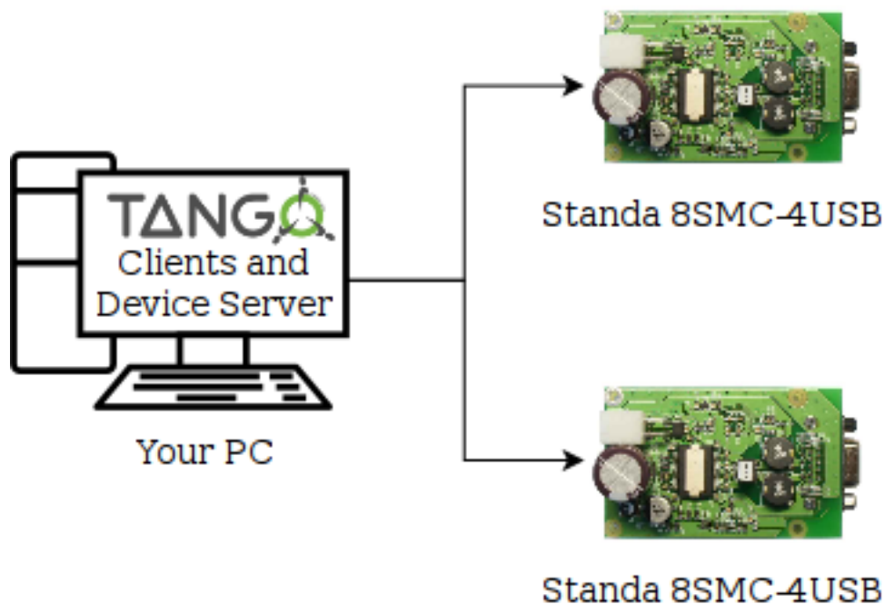
Рис. 4.76: Использование интерфейса TANGO через сервер устройств, запущенный напрямую на вашем ПК
