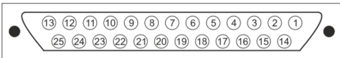
Рис. 4.29: Внешний вид и нумерация выводов разъёма DB-25 (вид спереди)
