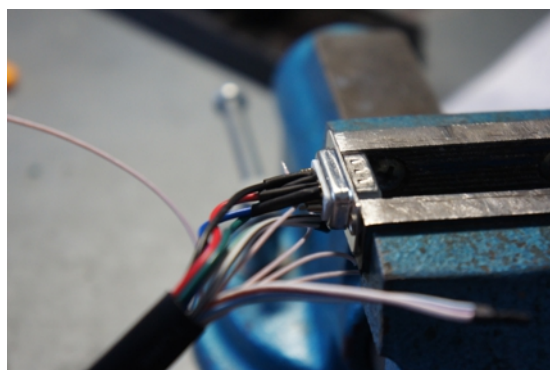
Рис. 3.17: Припаянные контакты обмоток мотора
