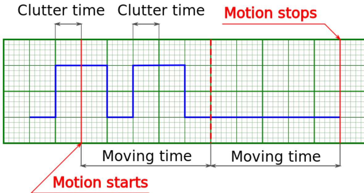
Рис. 4.54: Движение произойдёт один раз на двойное расстояние так как второй импульс синхронизации сработал до окончания первого движения
