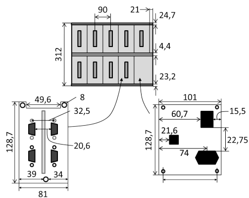
Многоосная система. Вид сзади. Со стороны силового разъёма 220В и модулей с контроллерами.
