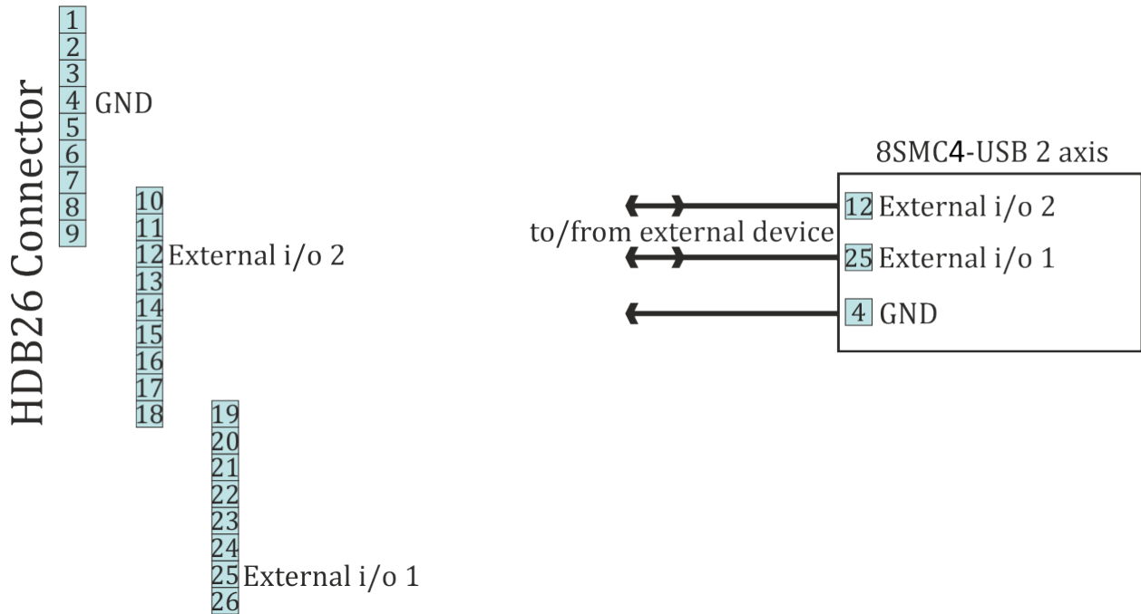
Рис. 4.67: Схема подключения к цифровому входу-выходу в двухосной системе
