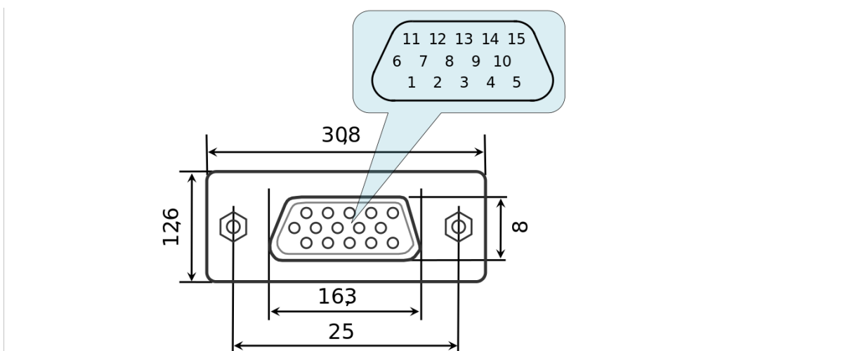
Рис. 4.18: Размеры и нумерация выводов в разъеме DSub, вид спереди
