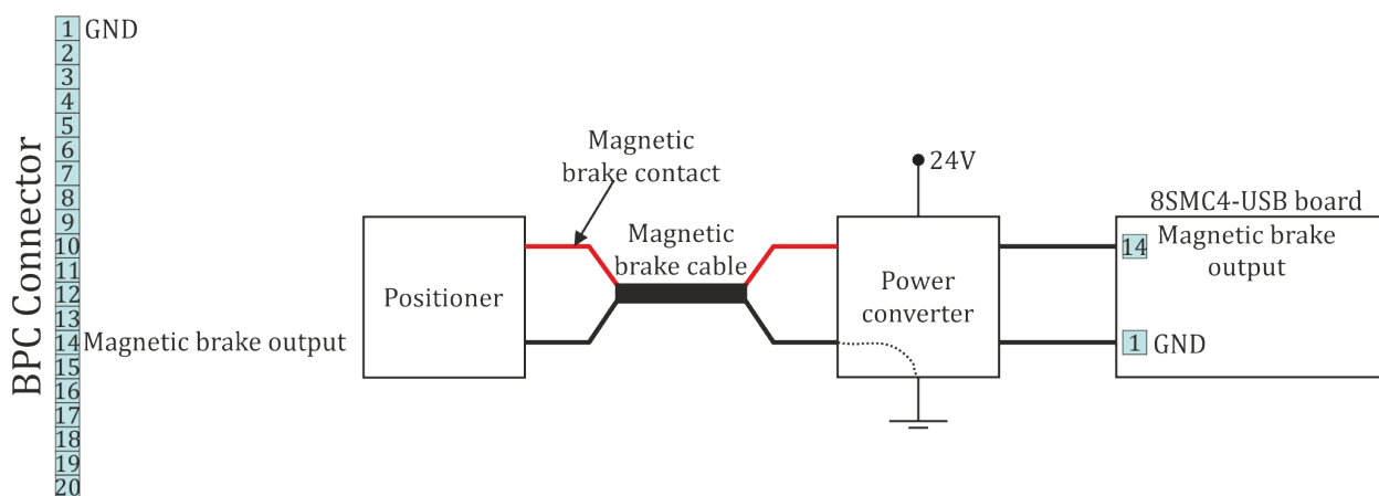
Рис. 4.41: Схема подключения магнитного тормоза к плате контроллера
