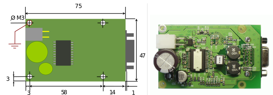
Контроллер. Вид сверху. Со стороны силового модуля и радиатора.
