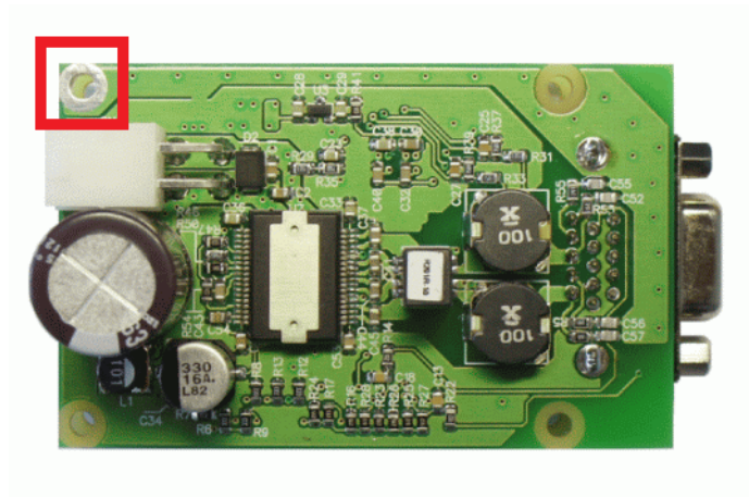
Рис. 2.1: Внешний вид платы контроллера сверху. Красным квадратом отмечена клемма заземления
