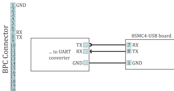
Рис. 4.71: Рекомендуемая схема подключения для платы контроллера
