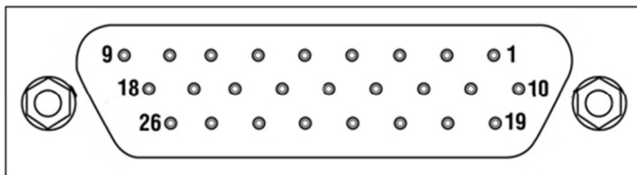
Рис. 4.23: Нумерация выводов в разъеме HDB-26, вид спереди
