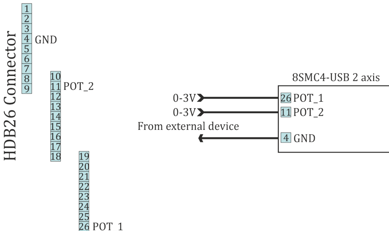
Рис. 4.69: Схема подключения к аналоговому выводу в двухосной системе
