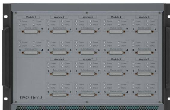
Рис. 4.27: Внешний вид передней панели
