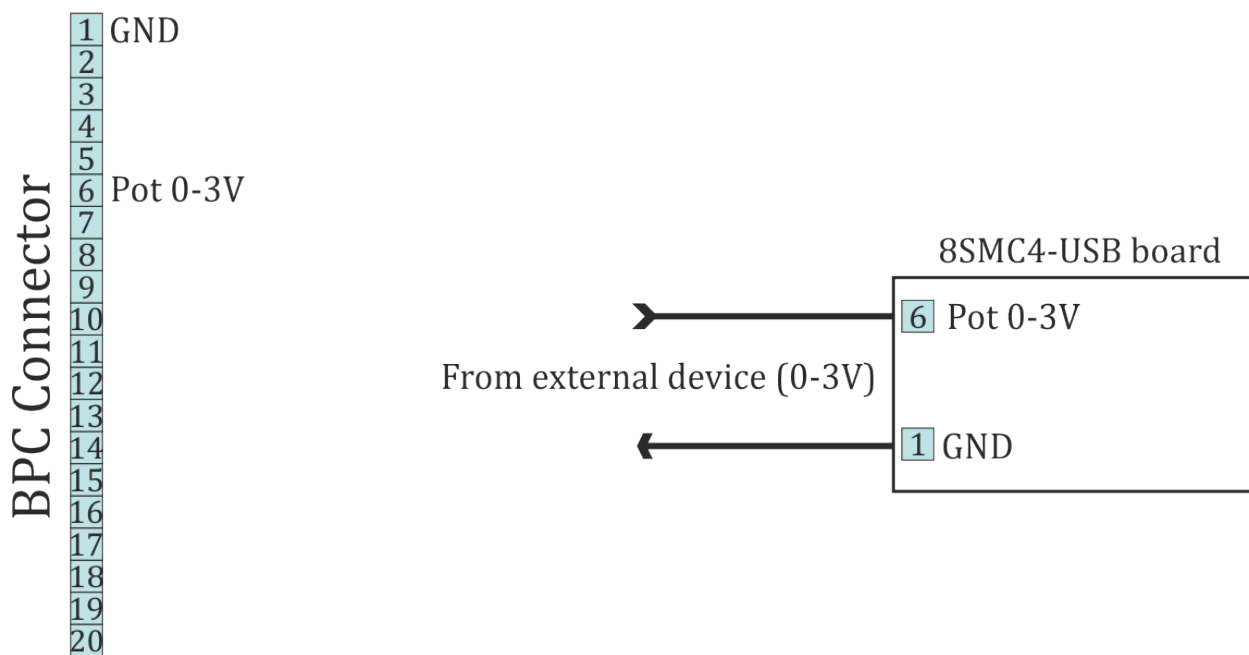
Рис. 4.68: Схема подключения к аналоговому выводу на плате контроллера
