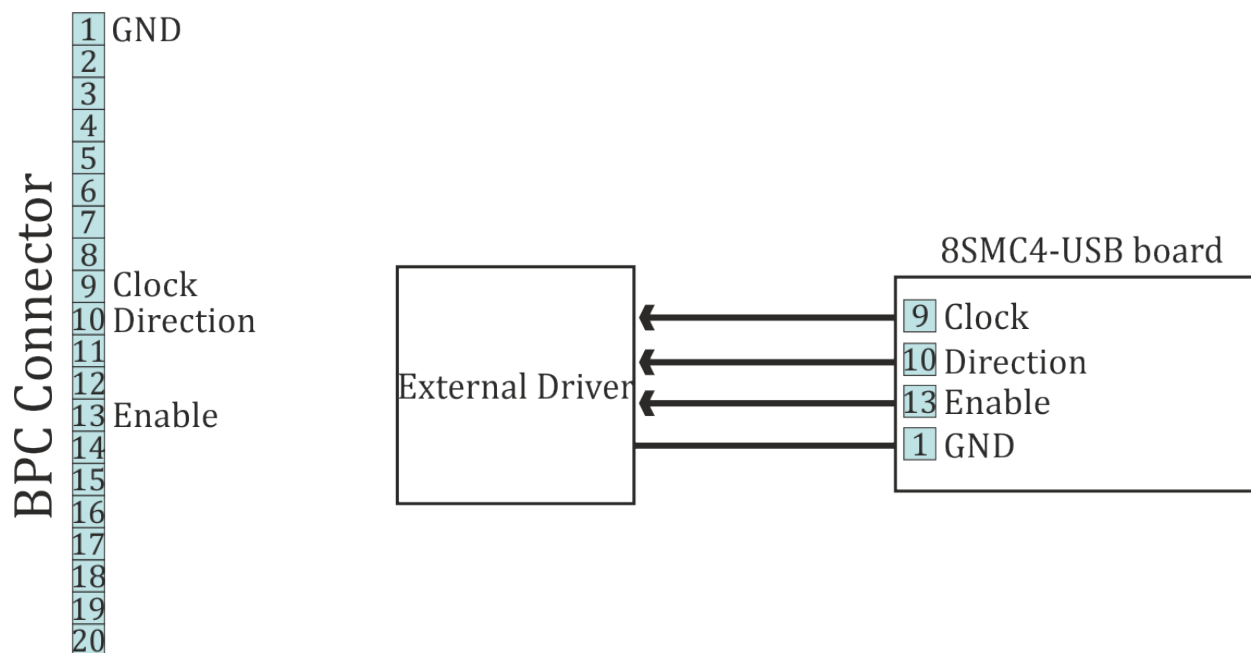
Рис. 4.70: Схема подключения к внешнему драйверу
