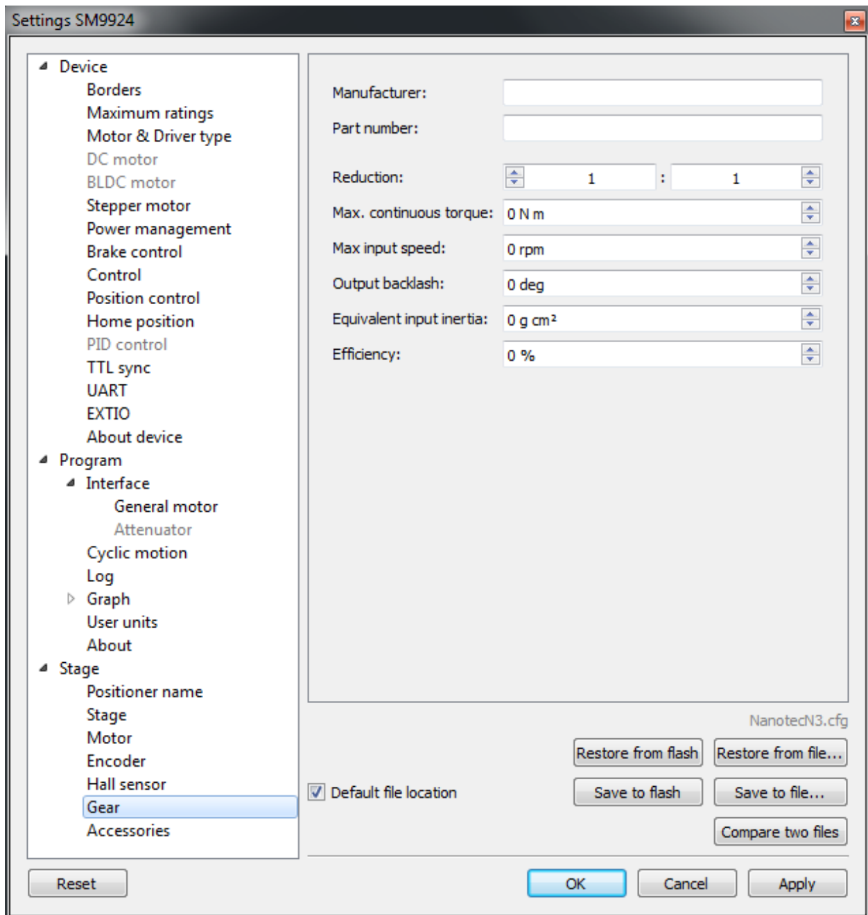
Рис. 5.52: Окно с описанием характеристик редуктора
