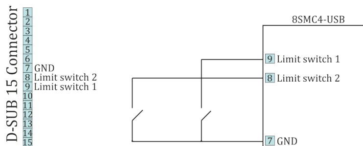
Рис. 4.31: Подключение концевиков типа «сухой контакт»
