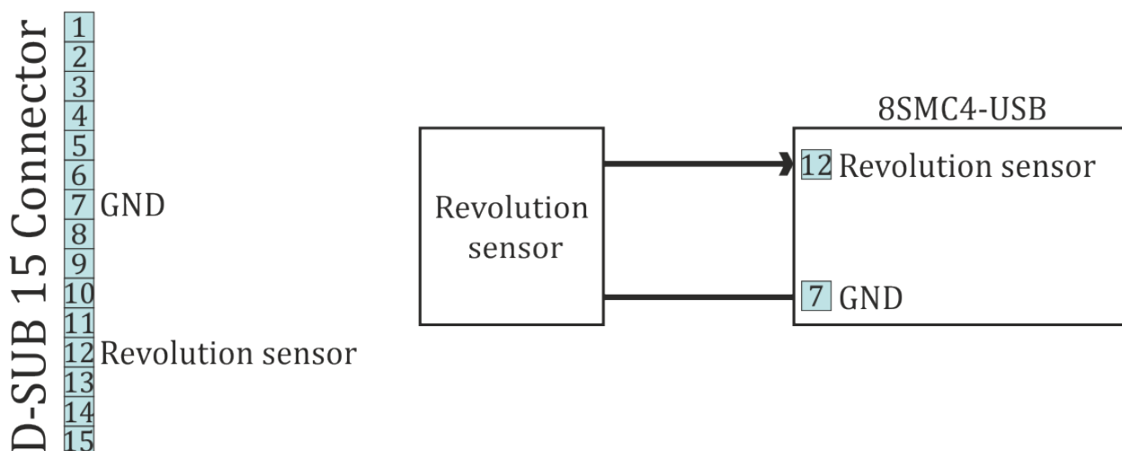
Рис. 4.36: Схема подключения датчика оборотов к системе на базе 8SMC4-USB
