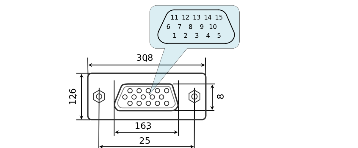
Рис. 4.25: Размеры и нумерация выводов в разьеме DSub, вид спереди
