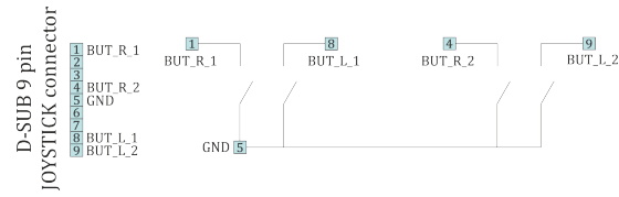
Рис. 4.48: Схема подключения кнопок к разъёму двухосной системы
