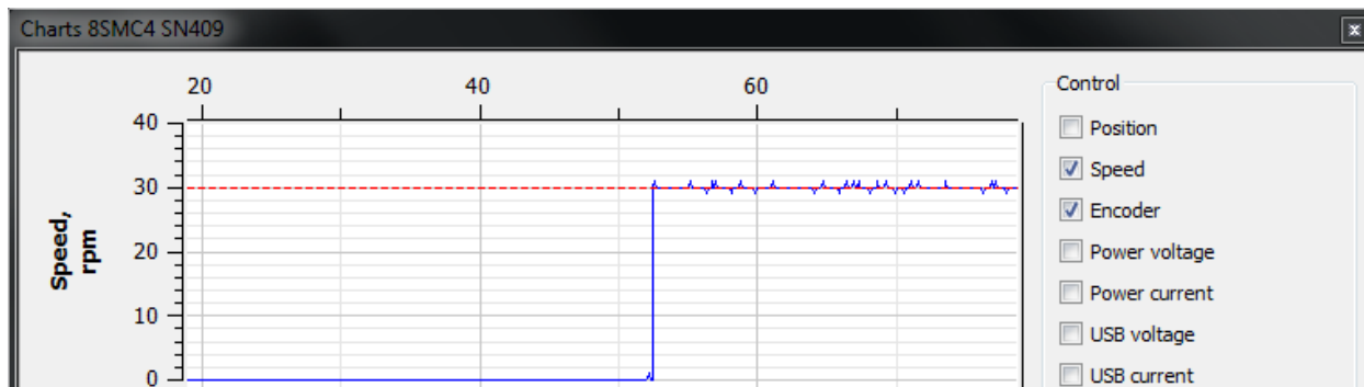
Рис. 5.18: График скорости в программе XiLab с ограничением скорости
