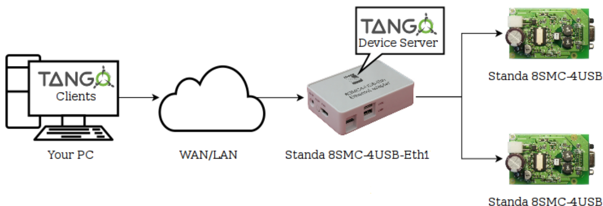
Рис. 4.77: Использование интерфейса TANGO через адаптер Standa 8SMC4-USB-Eth1
