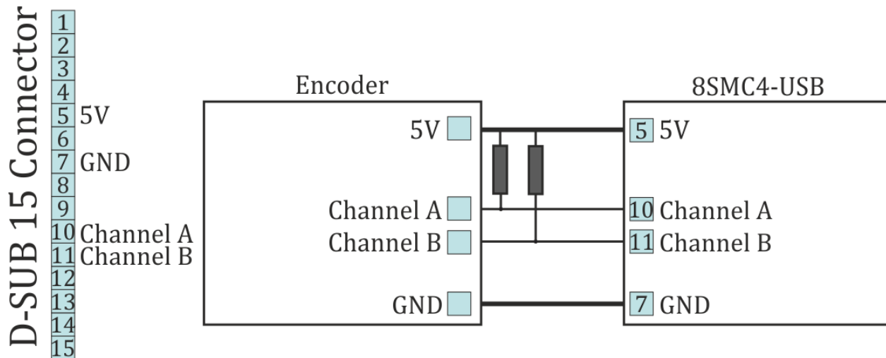
Рис. 4.34: Схема подключения простого энкодера к разъему DSub.
