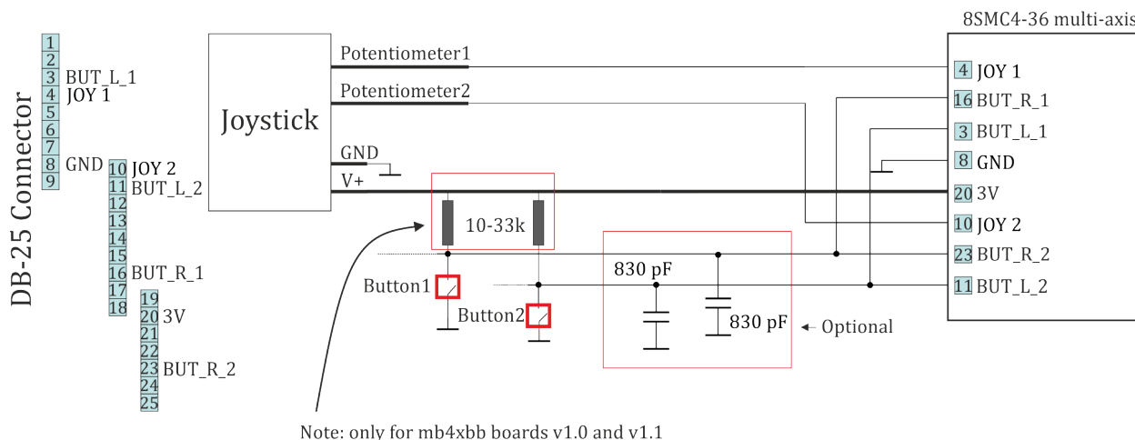
Рис. 4.46: Схема подключения джойстика к многоосной системе
