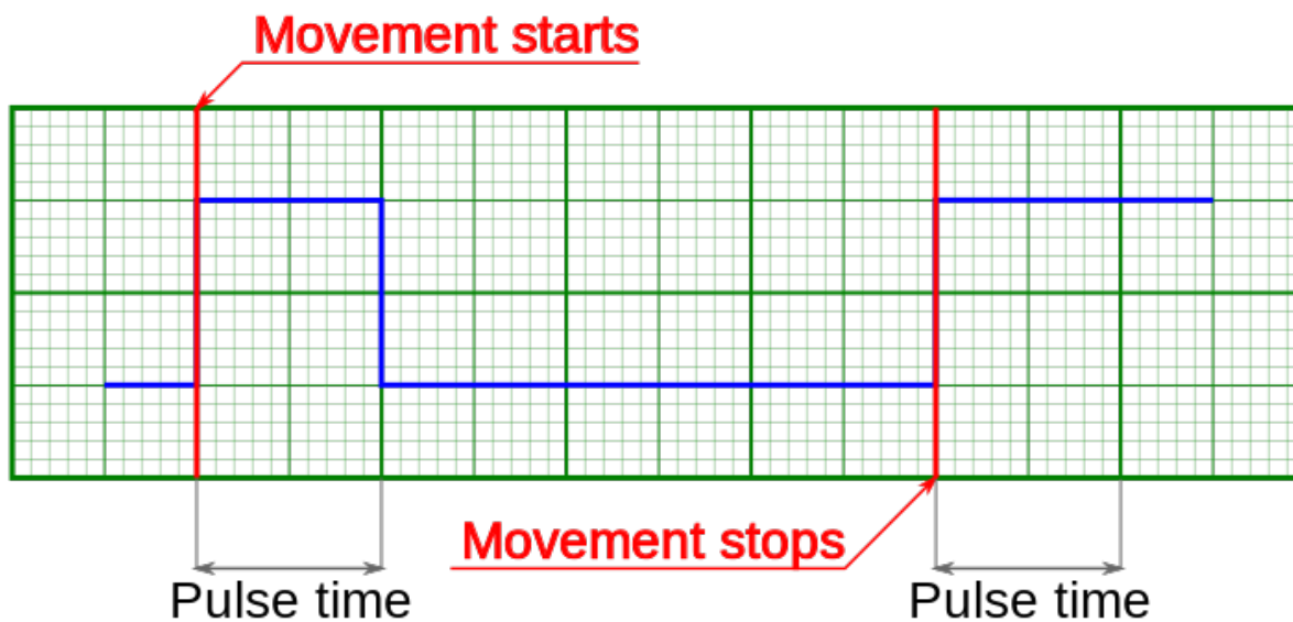
Рис. 4.57: Выходные импульсы синхронизации при генерации их на старте и на остановке движения (импульс измеряется в единицах смещения)
