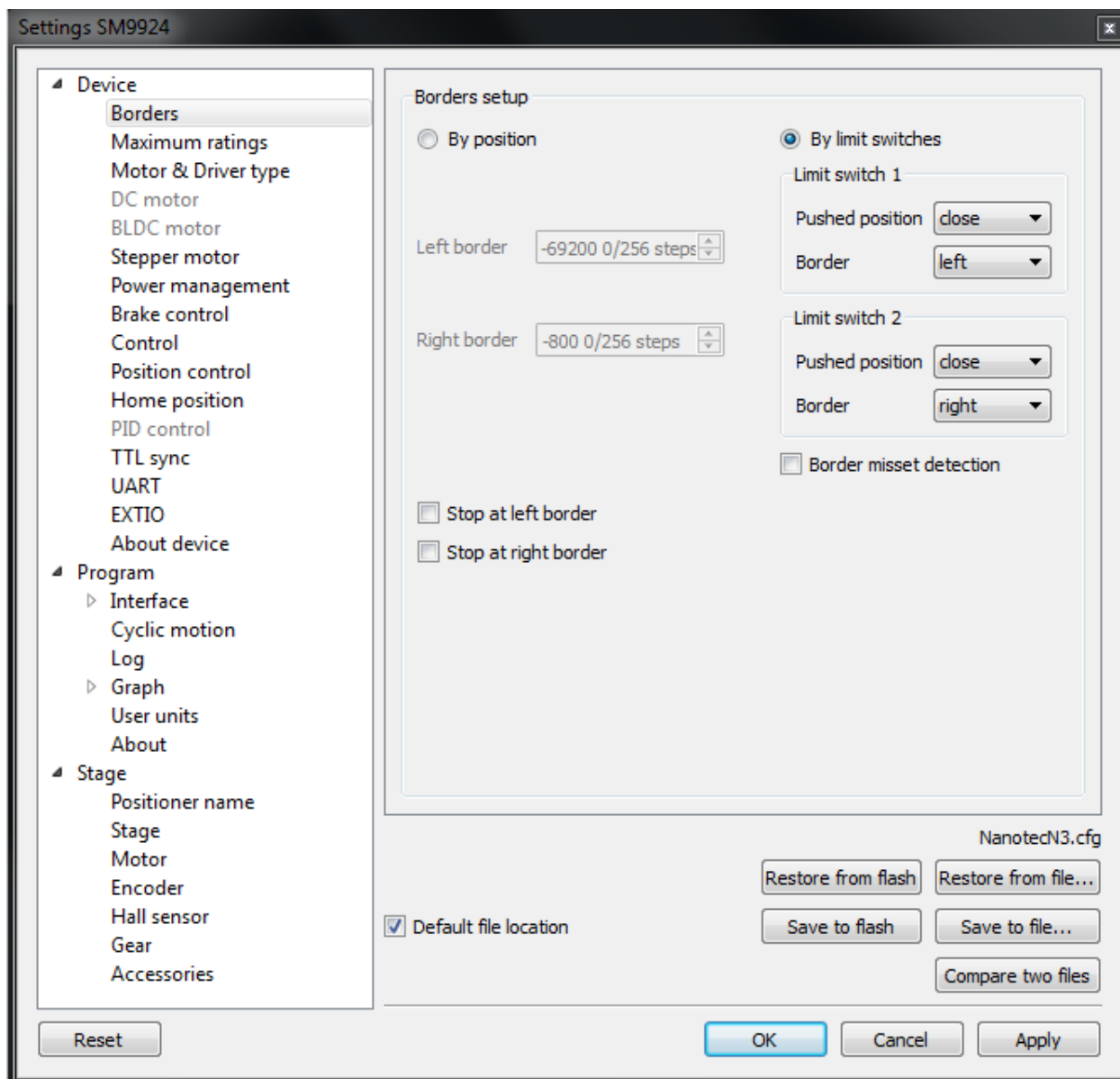
Рис. 5.22: Окно настроек диапазона движения и концевых выключателей
