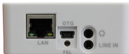
Рис. 7.4: Вид адаптера сзади. Слева направо: Ethernet разъём , mini-USB типа B , кнопка перехода в режим FEL , аналоговые вход/выход для микрофона и наушников
