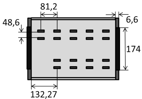
Многоосная система. Вид спереди. Со стороны передних разъёмов.
