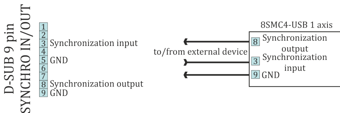
Рис. 4.62: Схема подключения к каналам синхронизации на одноосной системе
