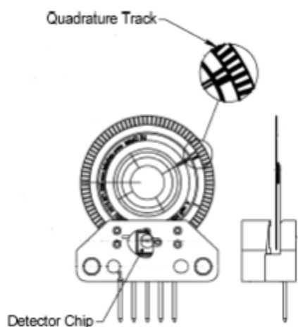
Рис. 4.33: Механика оптического квадратурного энкодера
