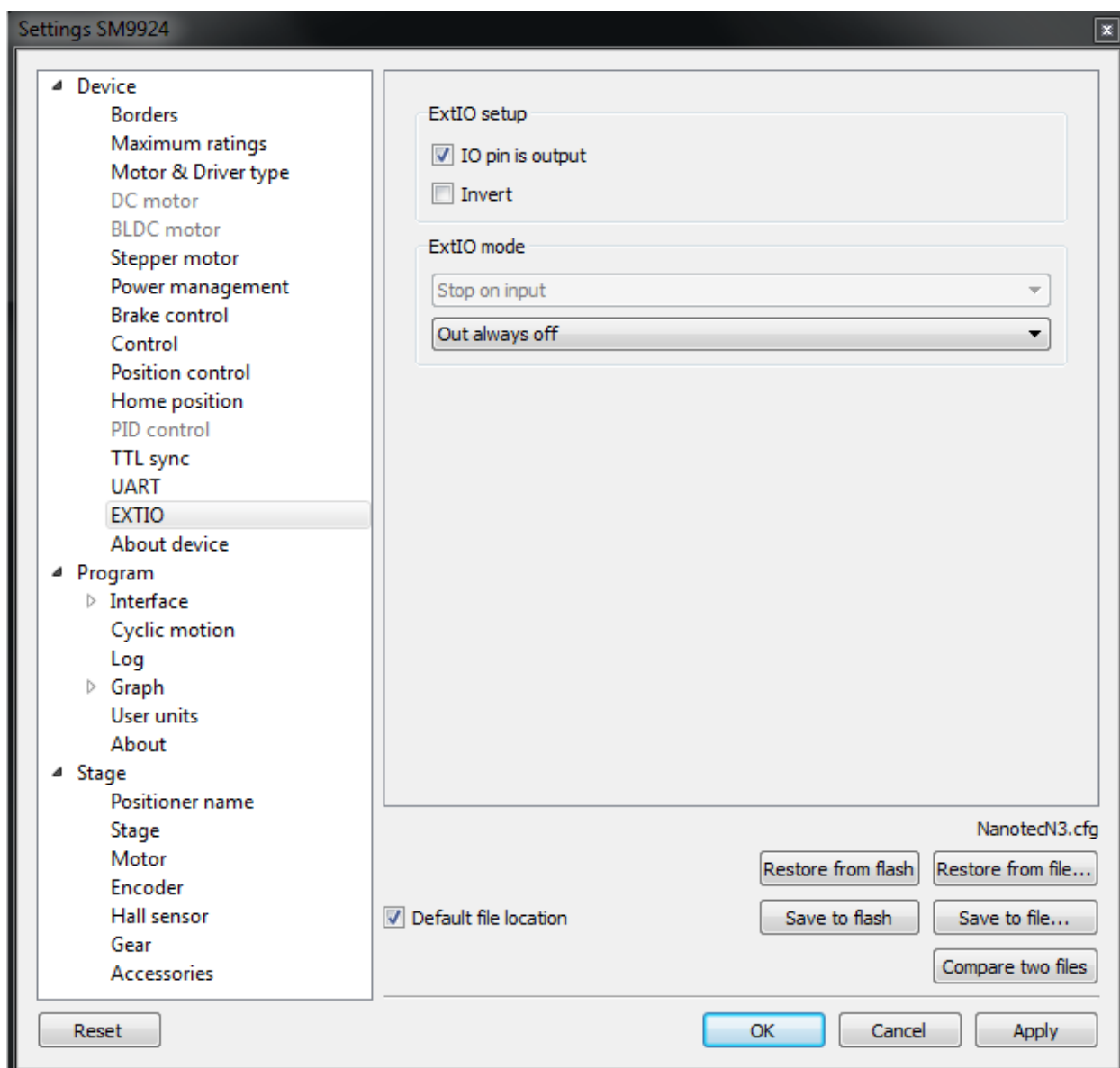
Рис. 5.31: Вкладка «Настройки цифрового входа-выхода общего назначения»
