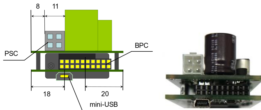
Контроллер. Вид сзади. Со стороны разъема для подключения к обводительной плате.
