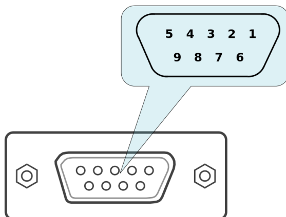
Рис. 4.14: Размеры и нумерация выводов в разъеме DSub, вид спереди
