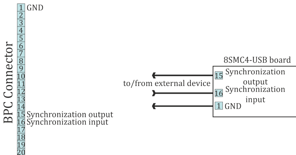
Рис. 4.61: Схема подключения к каналам синхронизации на плате контроллера
