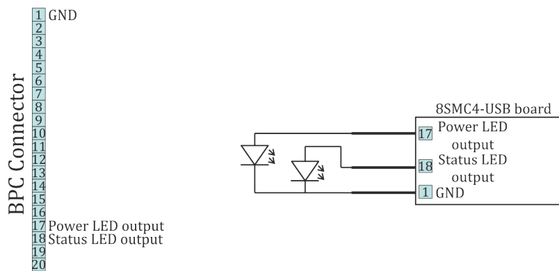
Рис. 4.38: Схема подключения индикаторов Power и Status к плате контроллера
