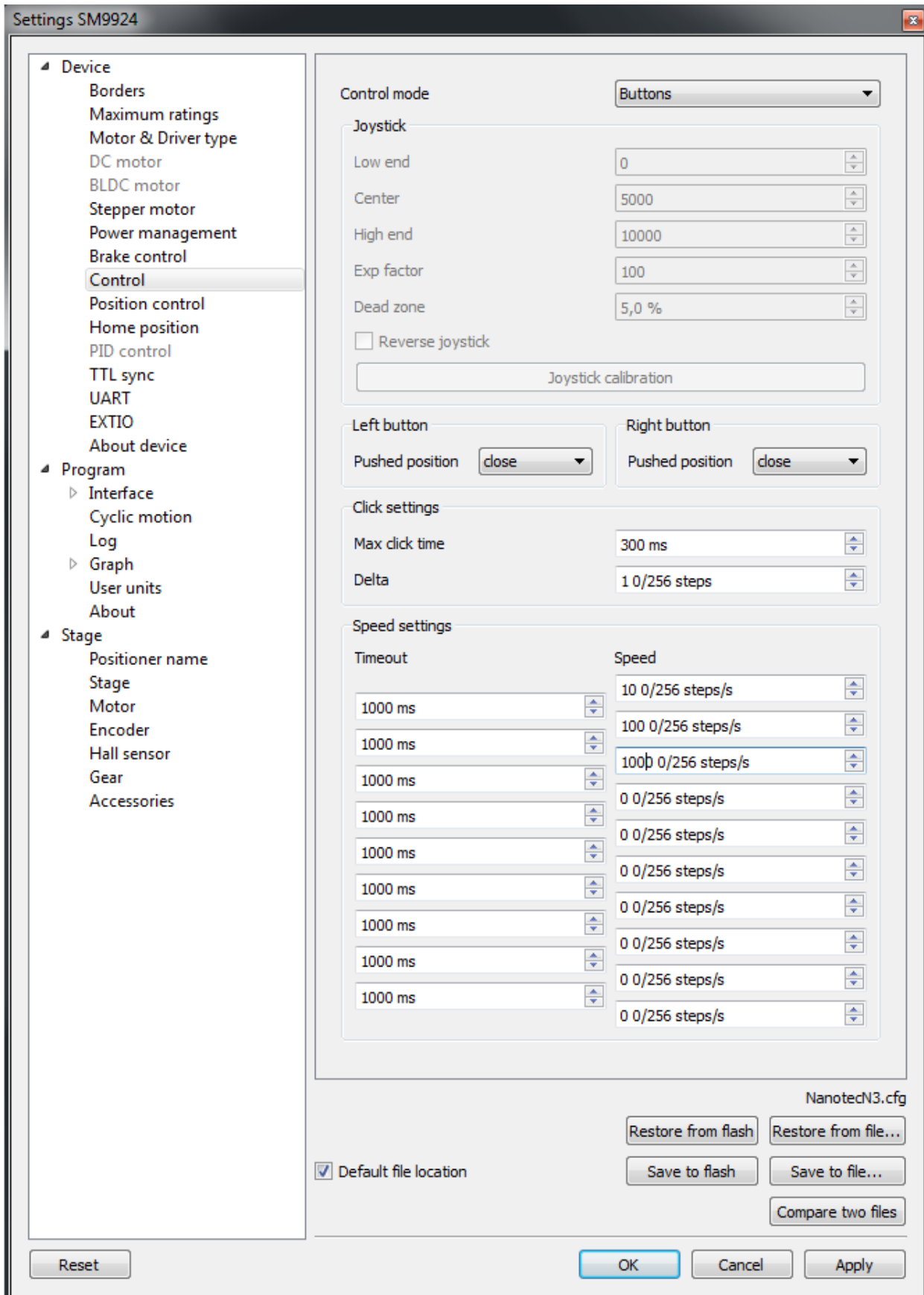
5.3. Настройки контроллера: Вид 5.30: Окно настроек внешних управляющих устройств
