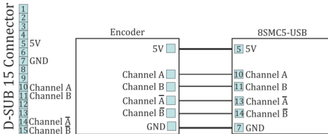
Рис. 4.35: Схема подключения дифференциального энкодера к разъему DSub.
