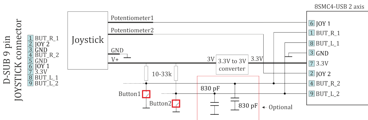
Рис. 4.45: Схема подключения джойстика к двухосной системе в корпусе через разъём D-SUB9
