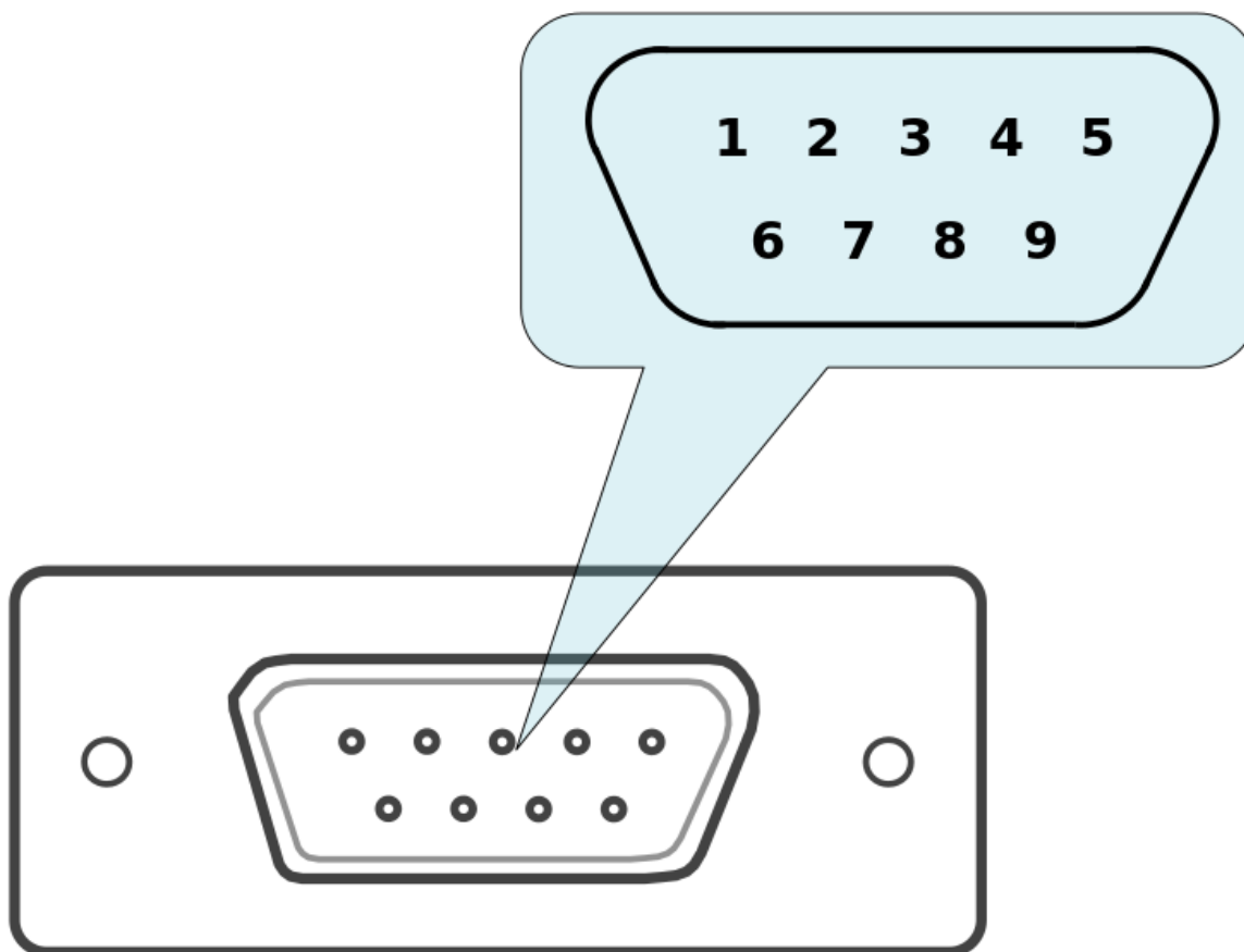
Рис. 4.21: Размеры и нумерация выводов в разъеме DSub, вид спереди
