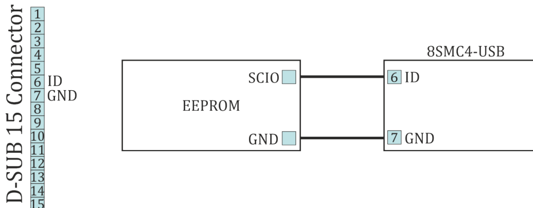
Рис. 4.73: Схема подключения для проверки внешней памяти
