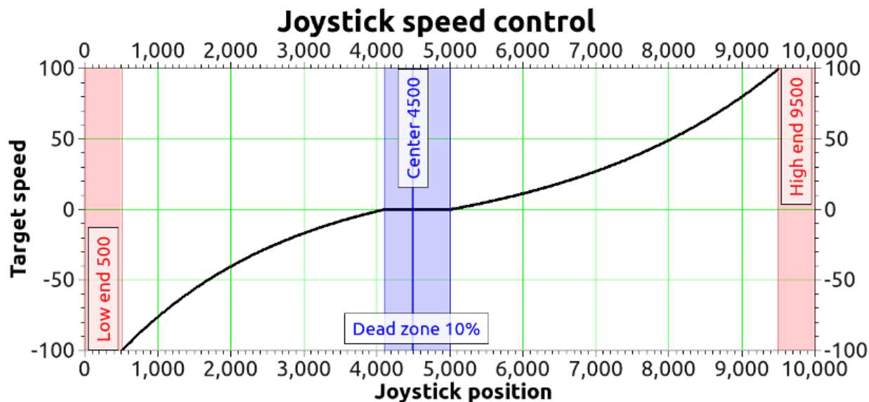
Рис. 4.43: Пример зависимости скорости движения от отклонения джойстика
