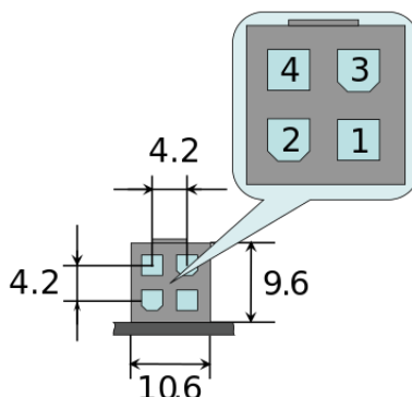
Рис. 4.3: Размеры и нумерация выводов в разьеме PSC (Power Supply Connector), вид спереди
