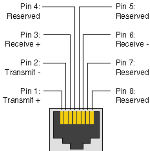
Рис. 4.26: Назначение выводов
